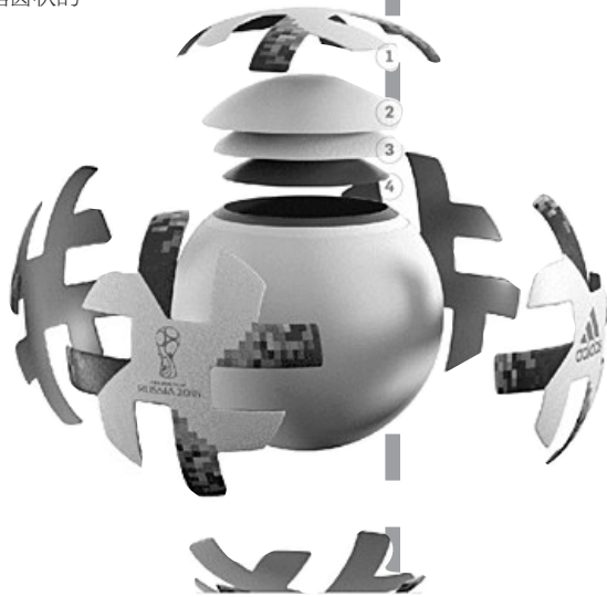
球的四层剖面图 (图片来自巴西媒体)
